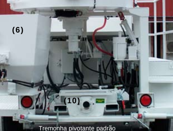
Tremonha pivotante padrão
